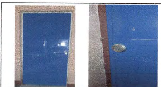
FOTO 6 : Mantenimiento a estructura (lijado, cambio de tubo , cepillado, sujeciones, aplicación de pintura) y Sustitución de chapa en aulas y Sustitución de chapa modulo de aula
